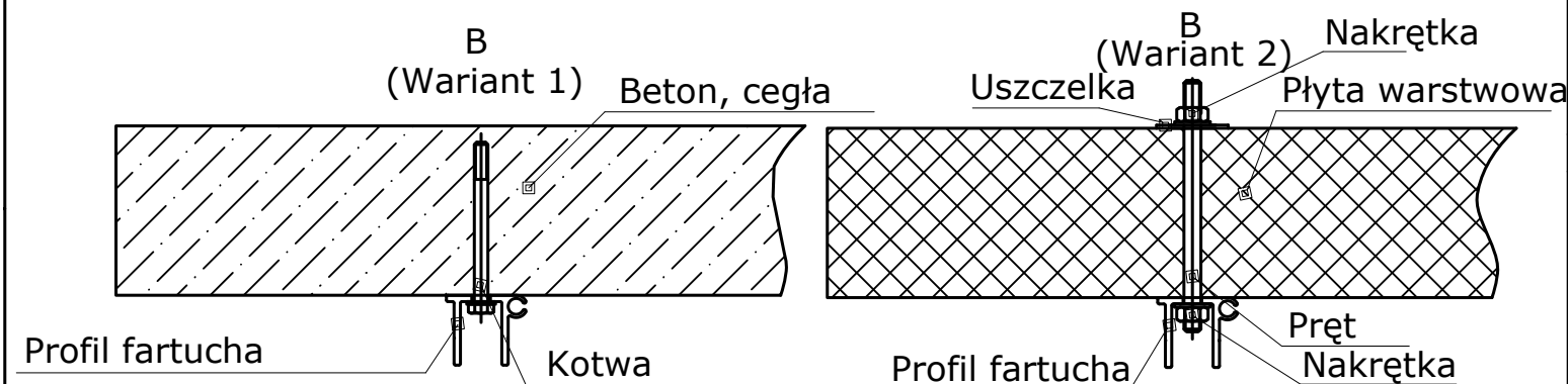
Rysunek przedstawia montaż standardowego fartucha uszczelniającego o wysokości 3400 mm i szerokości 3400 mm, (wysokość posadzki hali 1200mm)
